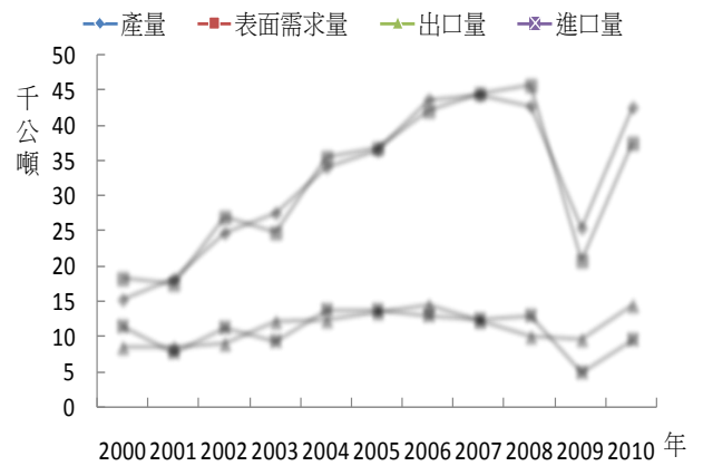
圖 9 台灣不銹直棒材供需分析
