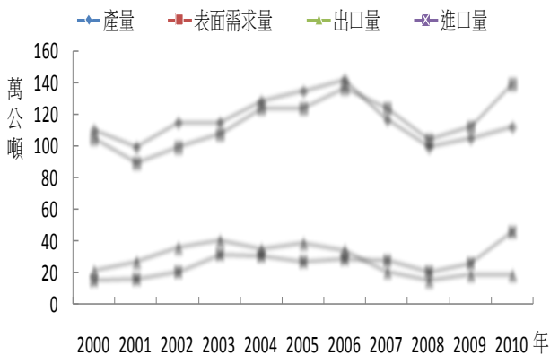
圖 6 台灣熱軋不銹鋼材供需分析
