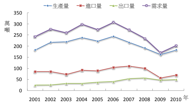
圖 4 美國不銹鋼材供需分析
