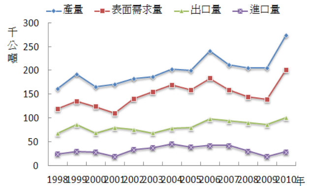
圖 8 台灣不銹盤元材供需分析
